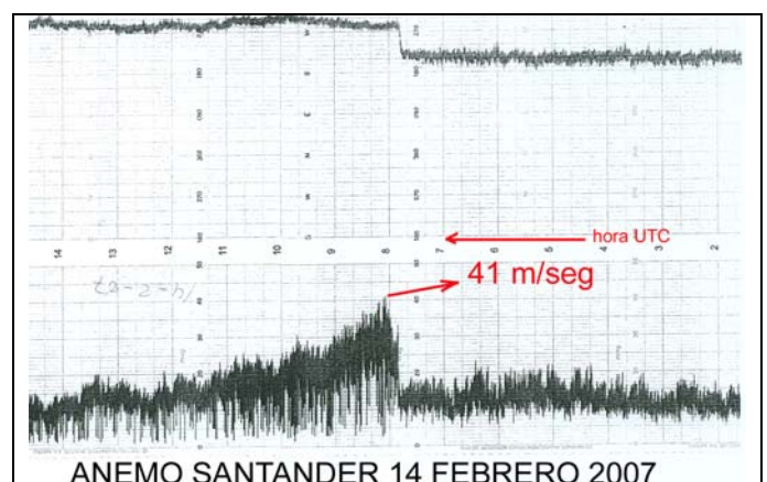
Fig. 2: Banda del anemo de Santander
